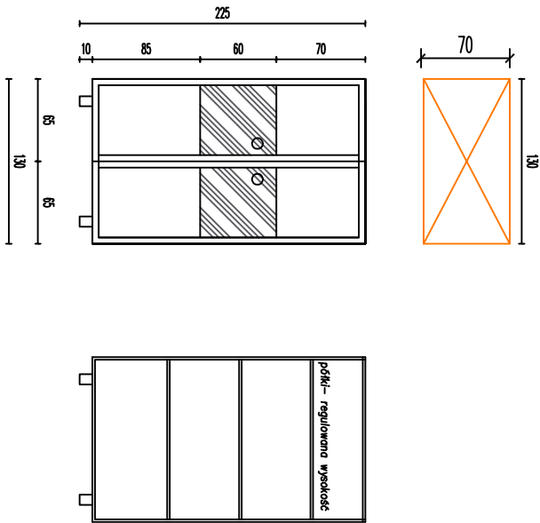
Szafa na pościel SZPOL
