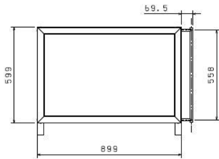
Top view Scale: 1:10
