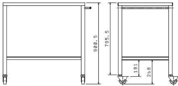
Front view Scale: 1:10
