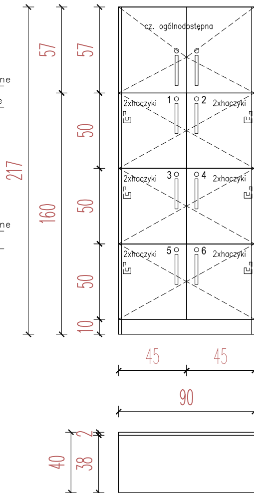
szafki na rzeczy osobiste z kluczykami i numerkiem szafki oznaczone numerem odpowiadającym kluczykowi numerki na szafkach z laminatu grawerskiego w kolorze stali szczotkowanej wysokość liter 3cm
