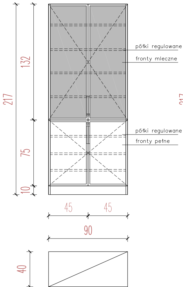
szafka magazynowa zamykana na klucz
