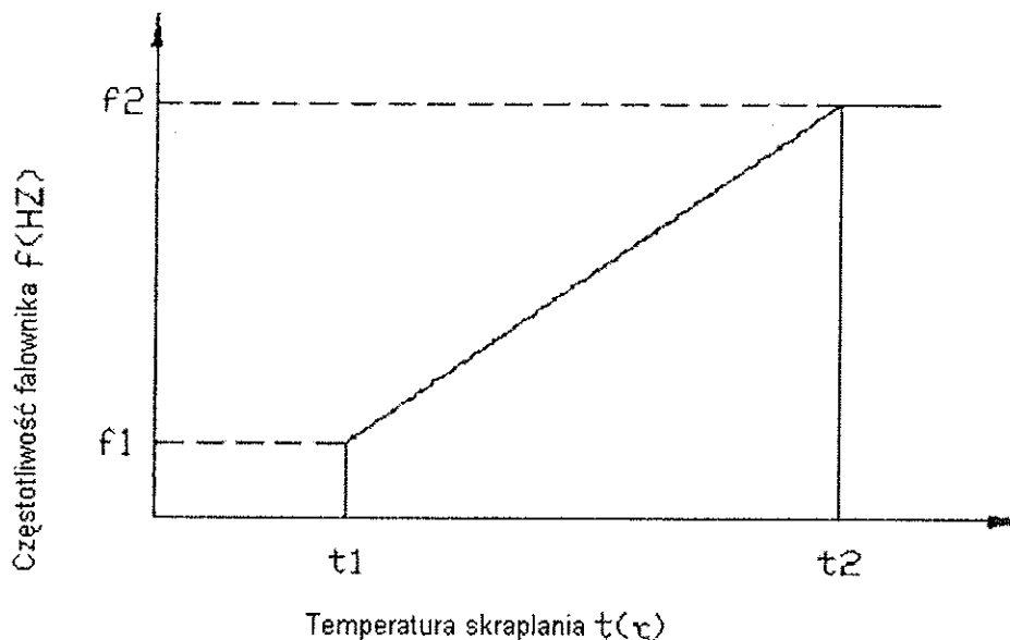
Rys. 1 Zależność między częstotliwością falownika a Temperaturą skraplania
