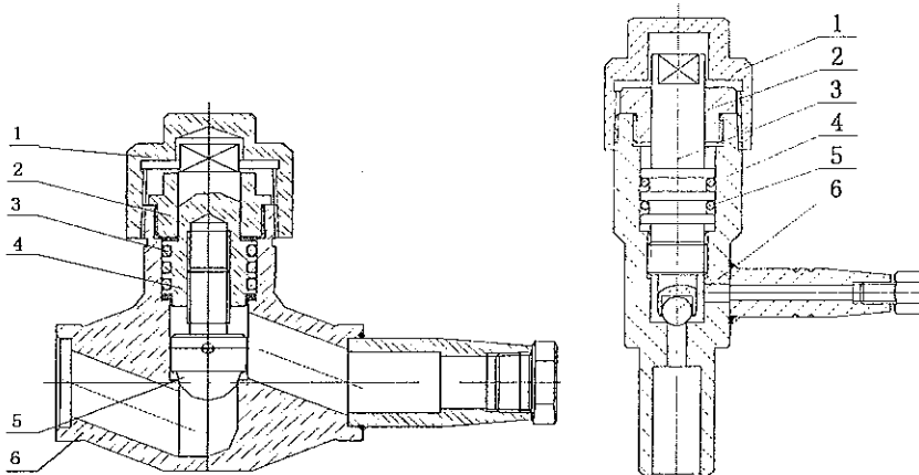
Rys. 6-5 Zawór zamykający typu DN10/II i DN25/II
