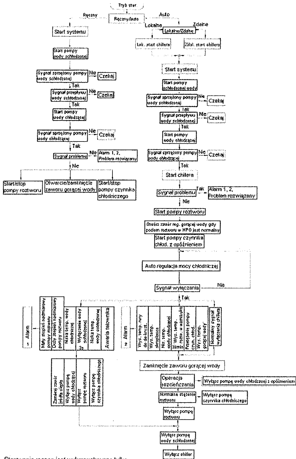
Rys. 4-4 Schemat Sterowania
