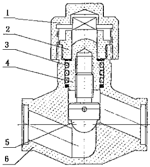
Rys. 6-4 Zawór zamykający typu DN10/1 i DN25/1
