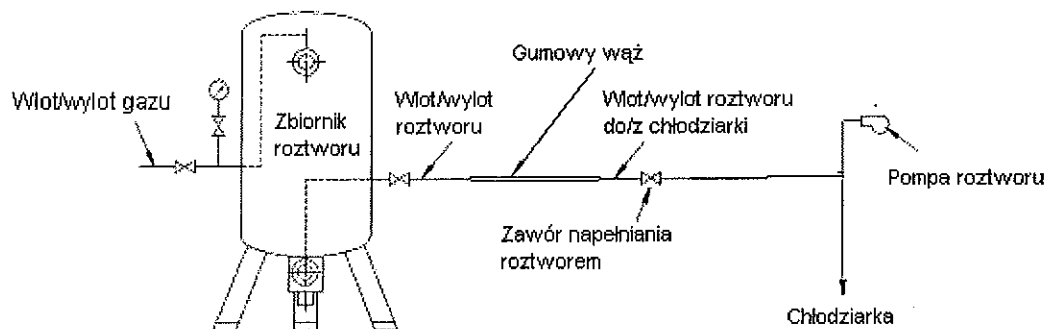
Rys 6-3 Przetłaczanie roztworu
