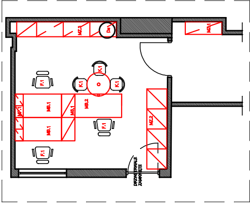
rzut pomieszczenia
