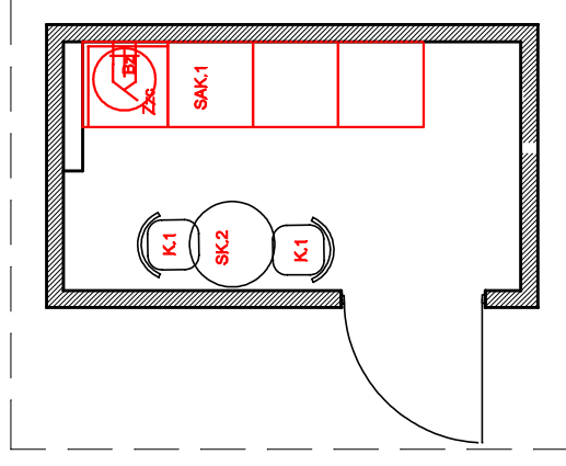
rzut pomieszczenia
