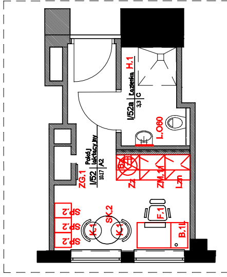
rzut pomieszczenia
